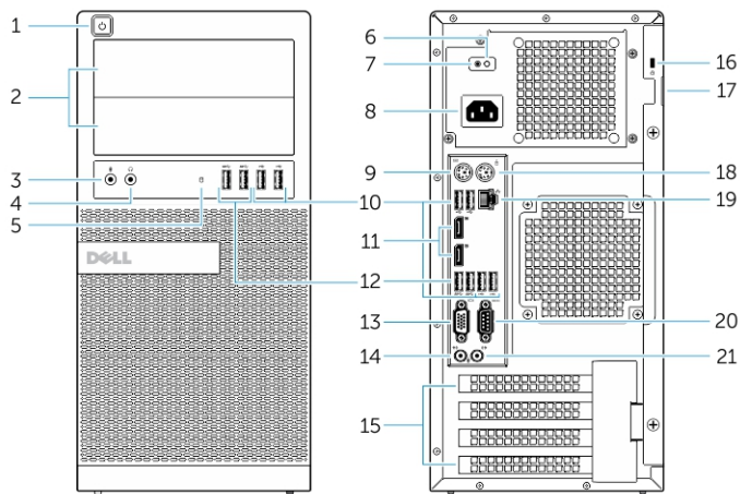
图 1: 小型塔式机的正面视图和背面视图
