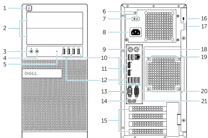
Skica 1. Pogled s sprednje in zadnje strani na mali pokončni računalnik
