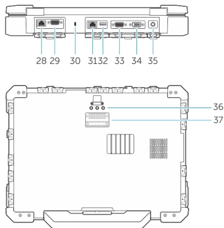
Рисунок 2. Вид системы сзади
