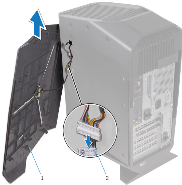
Рисунок 5. Снятие правой крышки
