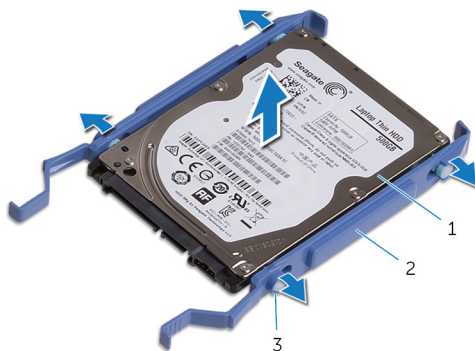
Рисунок 16. Извлечение жесткого диска из держателя
