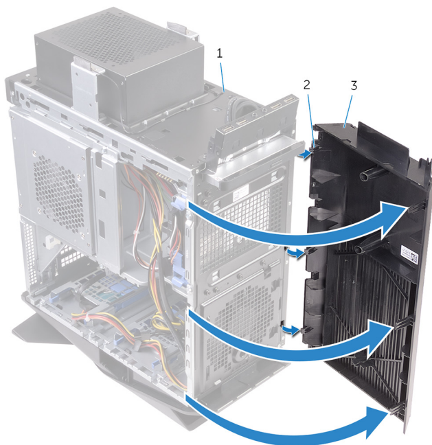
Рисунок 46. Снятие передней лицевой панели
